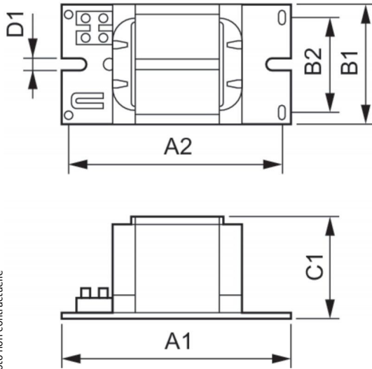
Ballast ferromagnétique BSN 400 K407-A2-ITS 230/240V 50Hz BC3
