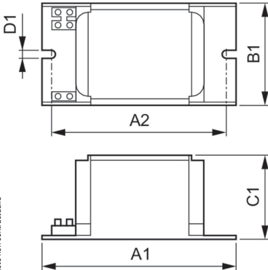
Ballast ferromagnétique BHL 250 K307-A2 230/240V 50Hz BC2-134
